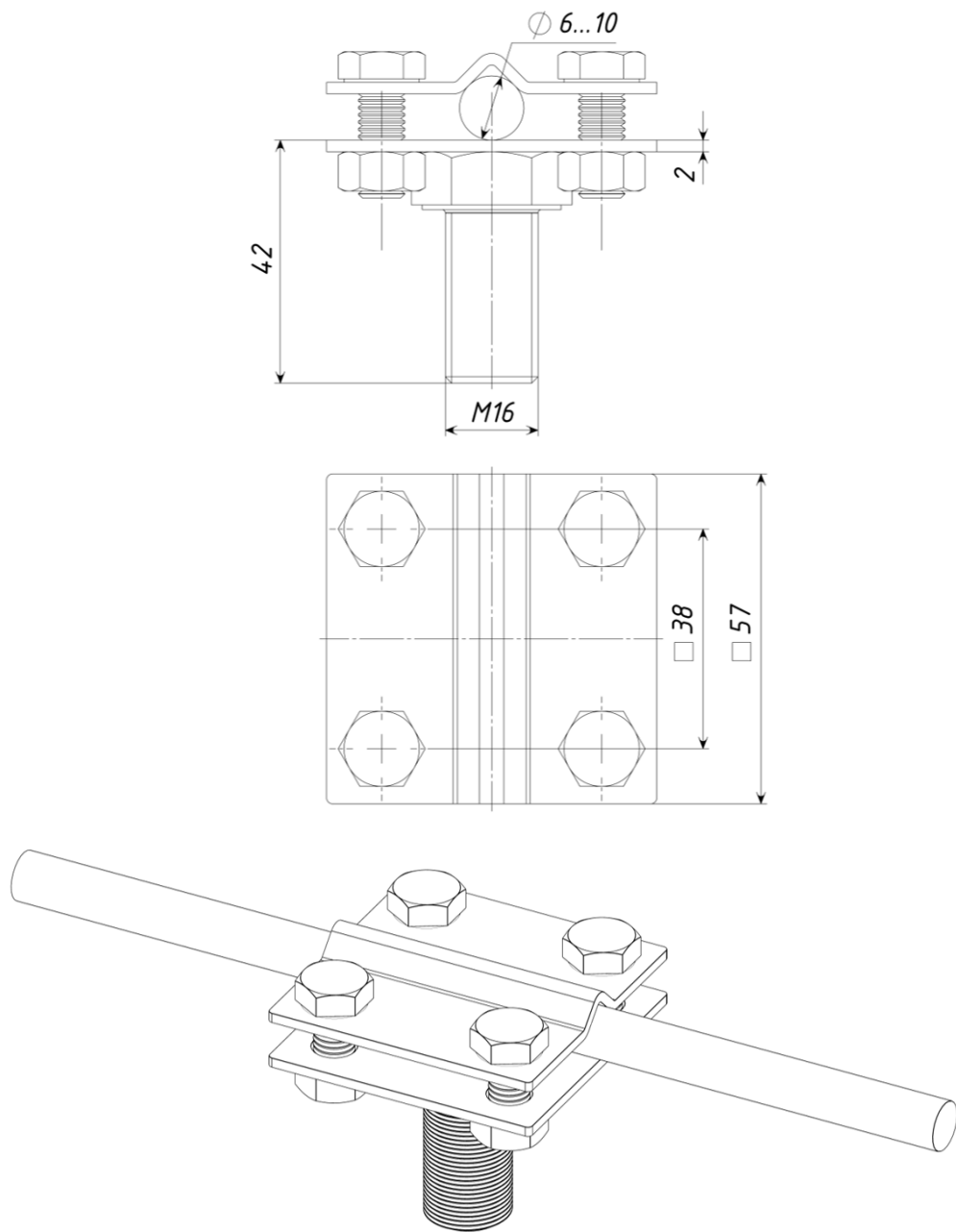
Рис. 1. Держатель-зажим фасадный прижимной LPS-037.
