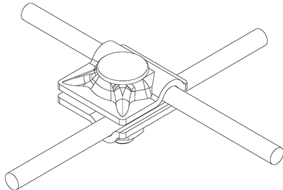
Рис. 3. Перпендикулярное соединение.
